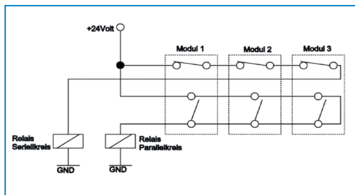
Schematische Darstellung der Stromkreise, gilt für Interlock und Notstopp
